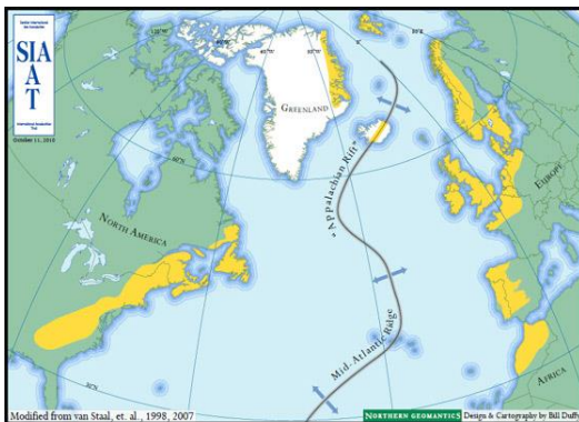
Distribución global de la geología apalachense
